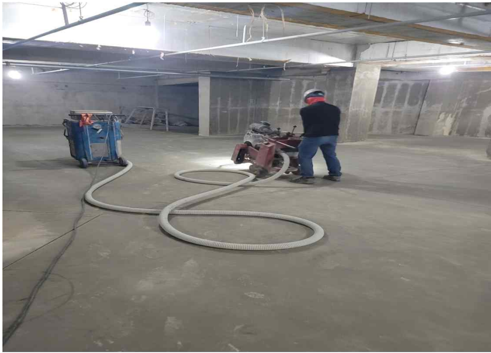
지하 주창장 누름 콘크리트 커팅작업
