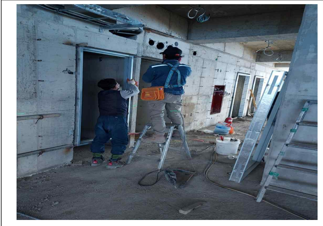
각 층 창호 프레임 설치
