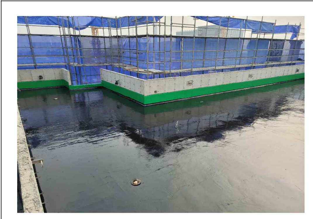
옥상 우레탄 방수작업
