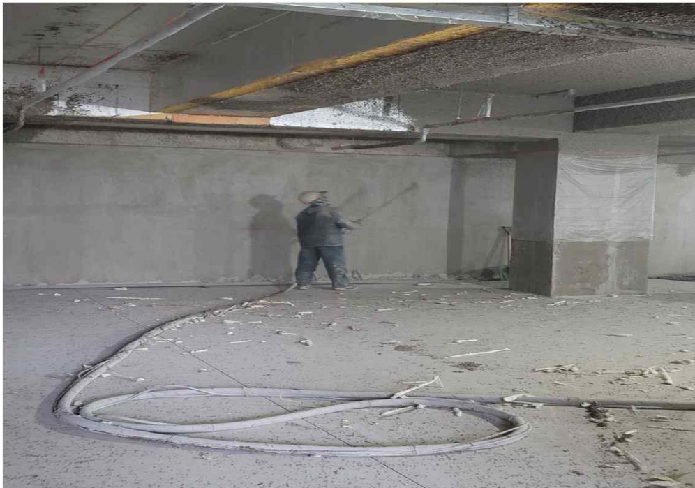
지하1층 천정 질석뿔칠공사
