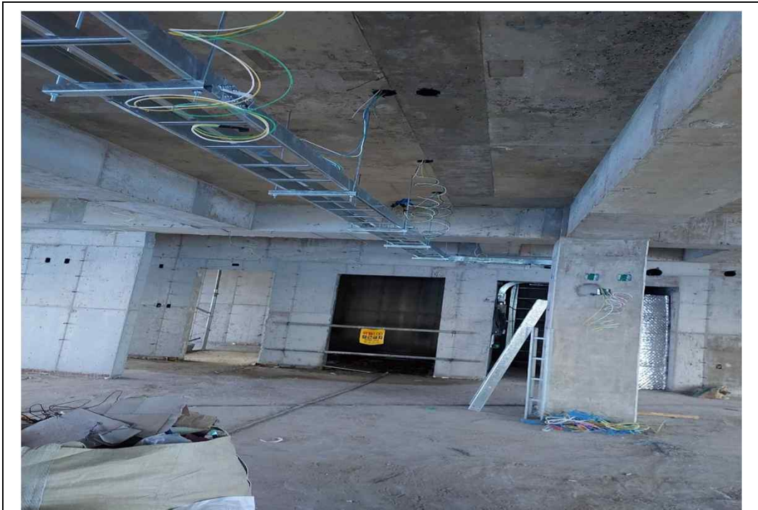
각 층 전기 트레이 설치
